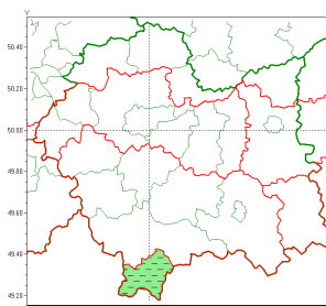
Opady śniegu 2020-02-04 08:46
