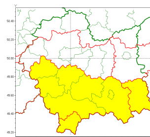
Zawieje/zamiecie śnieżne 2020-02-04 08:46
