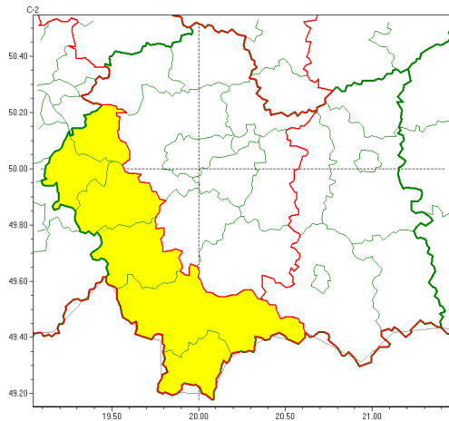
Burze z gradem 2022-08-25 05:27
