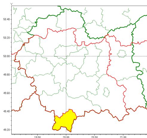
Opady śniegu 2020-02-03 23:20
