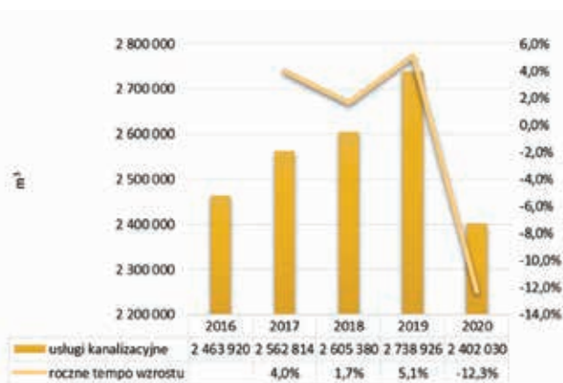
Porównanie ilościowe odbioru ścieków w latach 2016–2020 w m 3
